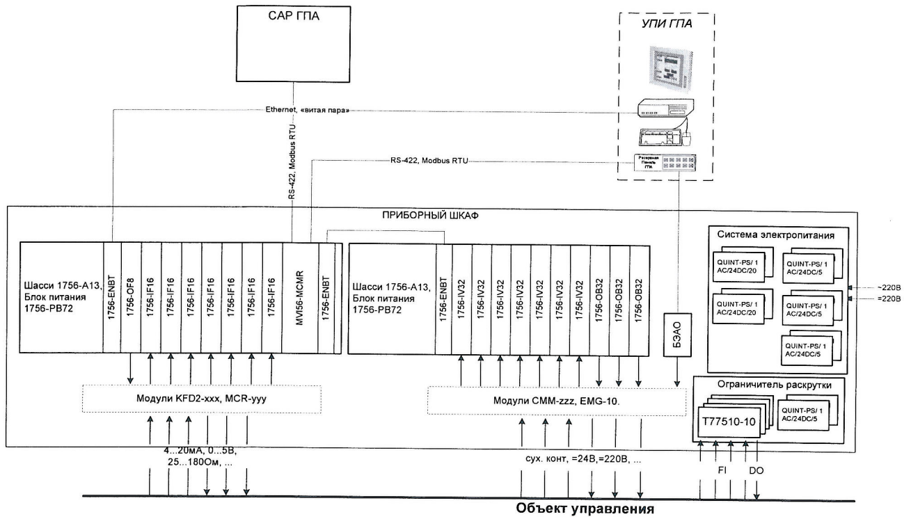
Рисунок 1. Структурная схема САУ ГПА после восстановительного ремонта
